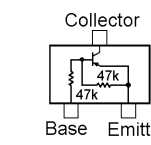
DTA144EM (16) (Q1036)
