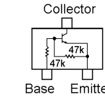
DTC144EM (26) (Q1031, 1039)
